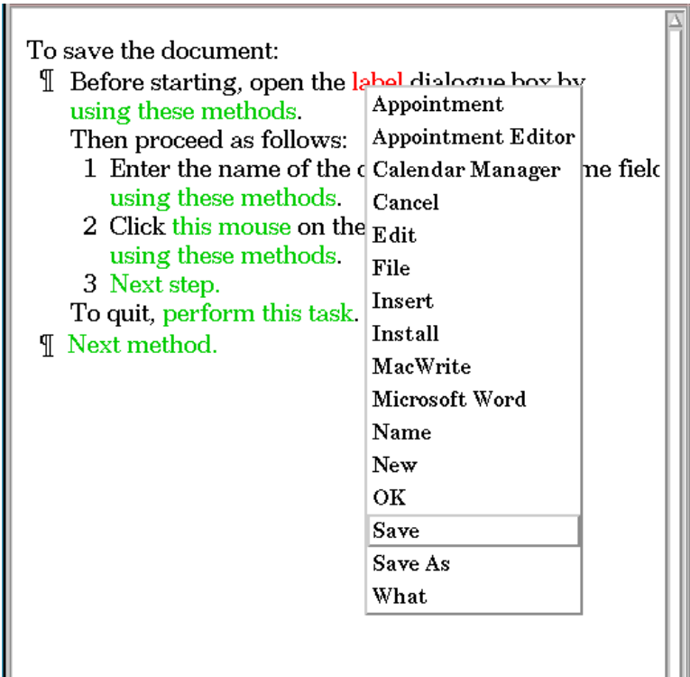
Fig. 9. WYSIWYM Editing.
