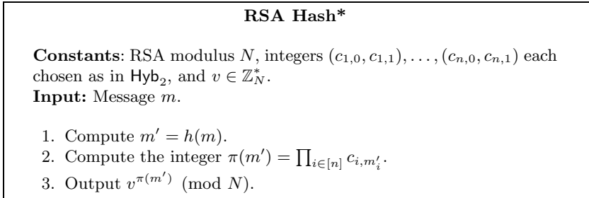
Fig. 4. RSA Hash*
