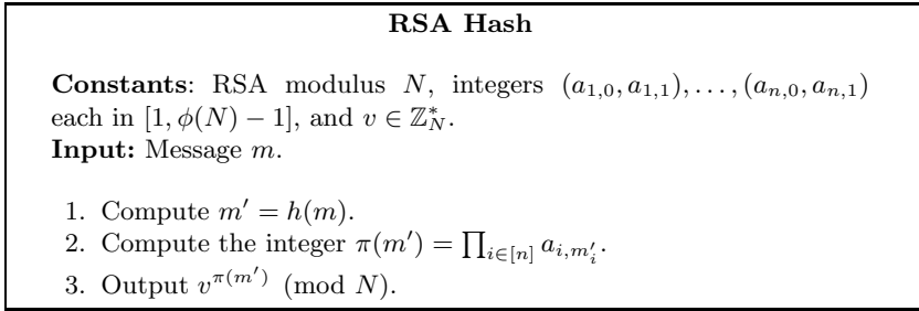
Fig. 3. RSA Hash
